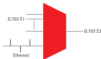
▼ MULTIPLEXING E1 CIRCUITS AND ETHERNET INTO E3
